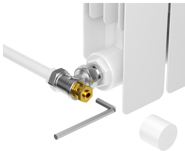
Настройка шестигранным ключом
