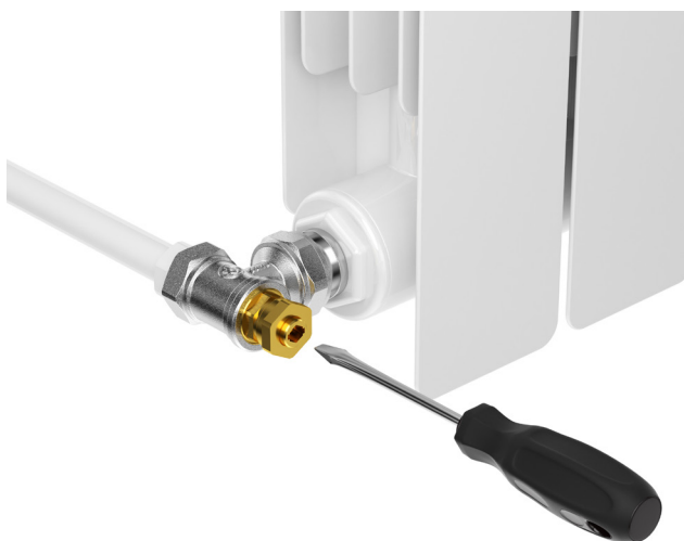
Настройка отверткой
